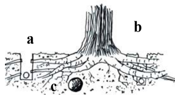
Fig.4: Paso de servicios “zanjas” por la zona de protección. A: zanja abierta en zonas alejadas. B: zanjas con “airspade” en proximidades tronco con elevada presencia de raíces. C: túnel en caso de pasar muy cerca o por debajo del árbol.
